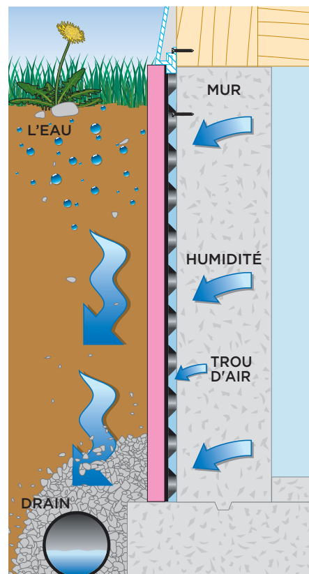
PLATON WRAP SUR MURS ISOLÉS
