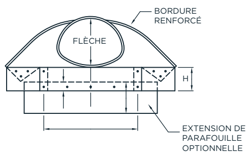
ÉLÉVATION
