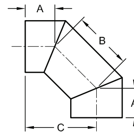
Coude à trois éléments 46° à 90°
