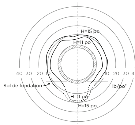
FIGURE 3B: RÉPARTITION DE LA CHARGE - TUYAU FLEXIBLE
