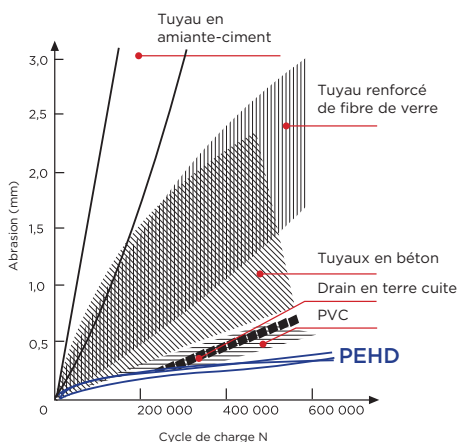
FIGURE 1: PERTE PAR ABRASION DES DIFFÉRENTS MATÉRIEAUX POUR TUYAUX*
