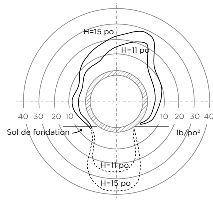
FIGURE 3A: RÉPARTITION DE LA CHARGE - TUYAU RIGIDE
