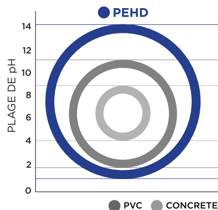
FIGURE 2: PLAGES DE pH DES MATÉRIEAUX DE TUYAUX DISPONIBLES SUR LE MARCHÉ
