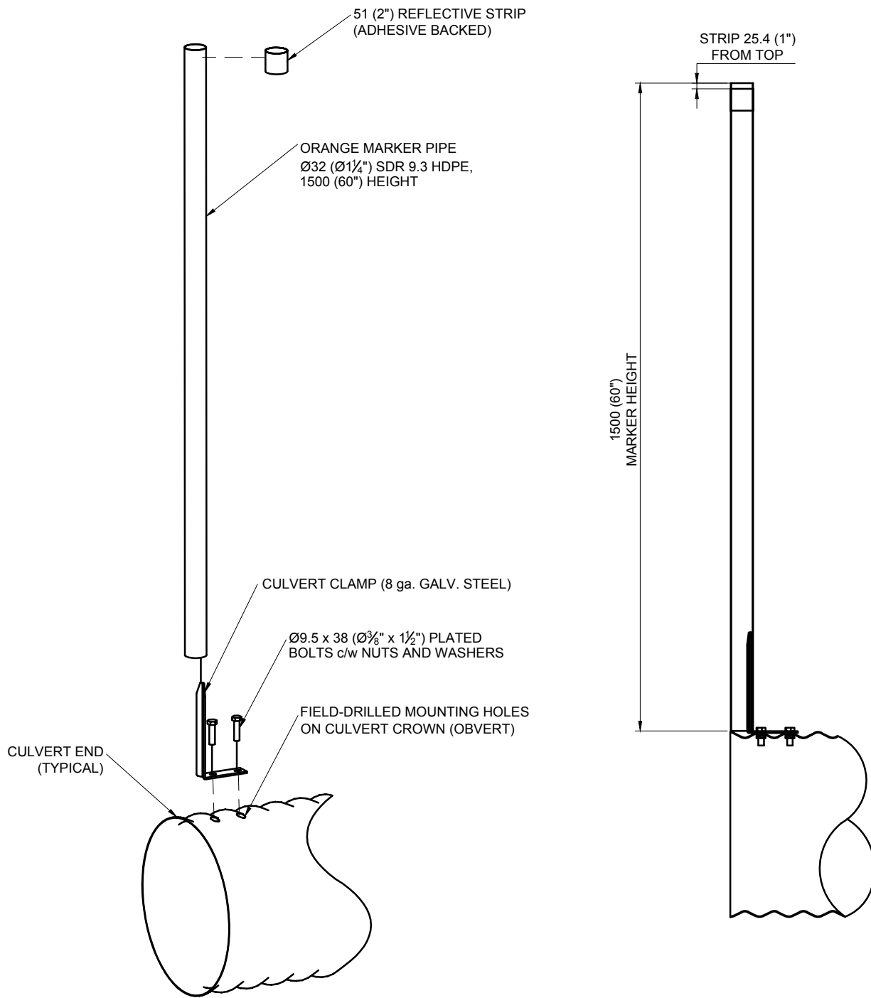
1 COMPONENTS CM-SD-01 SCALE N.T.S.
